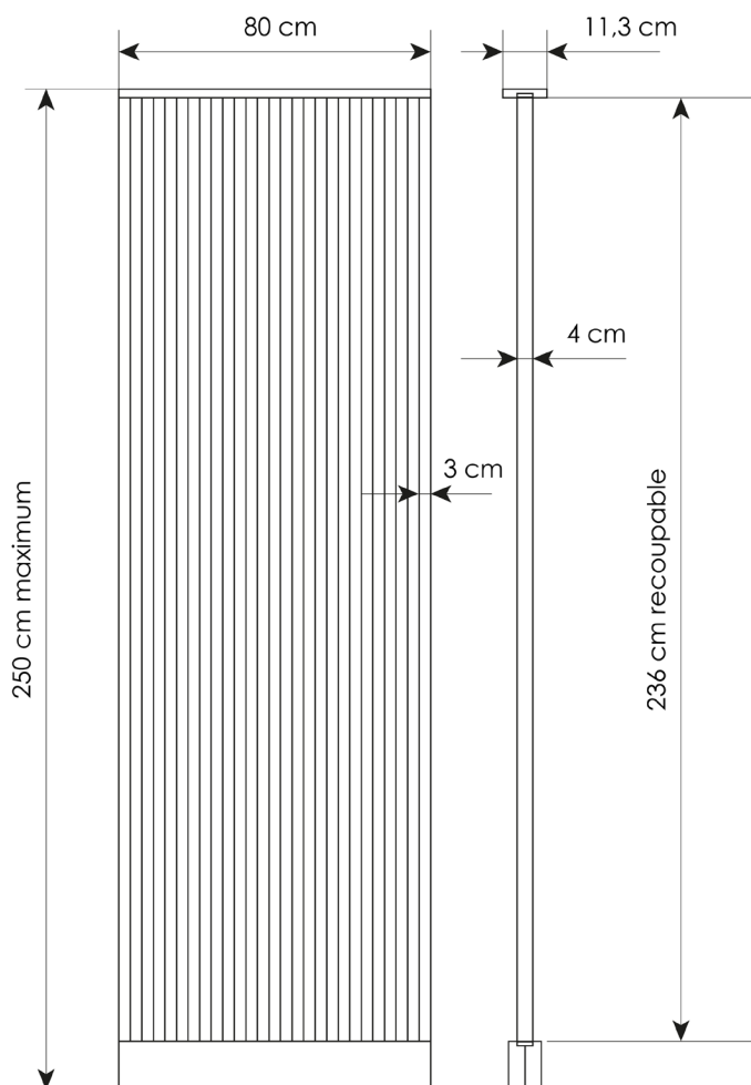
Visuel dimensions
