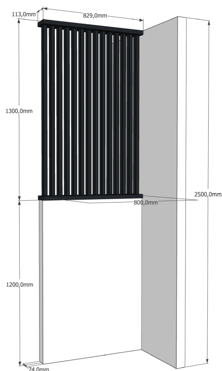
Visuel dimensions
