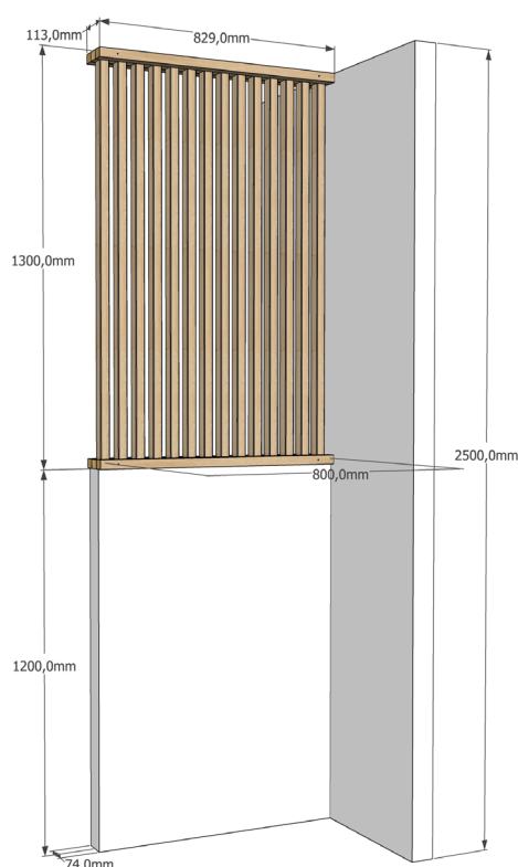
Visuel dimensions
